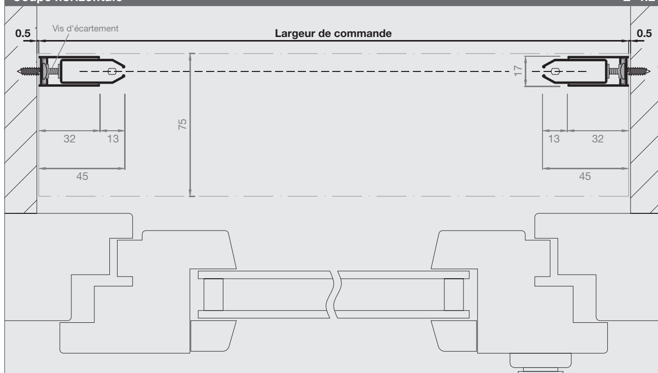
Coupe horizontale
